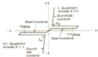
Bild 1 – Strom/Spannungs-Kennlinie (Prinzipdarstellung)
