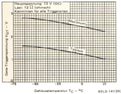
Bild 14 – Gate-Triggerspannung in Abhängigkeit von der Gehäusetemperatur
