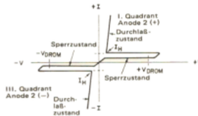
Bild 1 - Strom/Spannungs-Kennlinie (Prinzipdarstellung)
