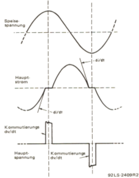
Bild 5 – Kommutierungs-Charakteristiken von Hauptstrom und -spannung
