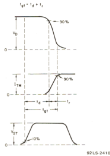
Bild 6 – Einschaltcharakteristiken
