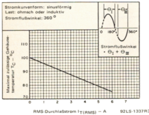
Bild 3 – Gehäusetemperatur in Abhängigkeit vom Durchlaßstrom
