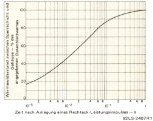
Bild 15 – Impulsärmewiderstand (Sperrschicht/Gehäuse) in Abhängigkeit von der Zeit
