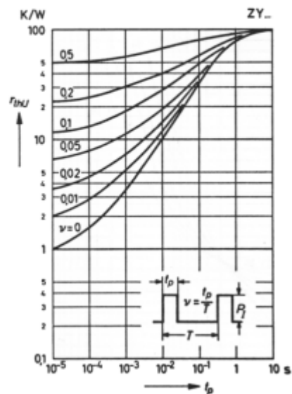
Impuls-Wärmewiderstand in Abhängigkeit von der Impulsdauer (siehe Fußnote 1) auf Seite 187)
