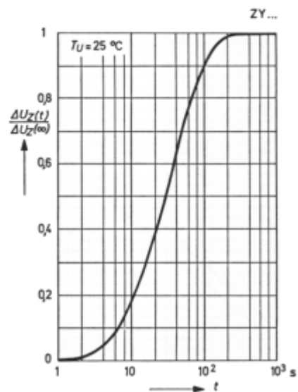
Änderung der Arbeitsspannung in Abhängigkeit von der Zeit nach dem Einschalten Relativwerte
